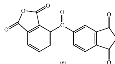
(6) a-BTDA
